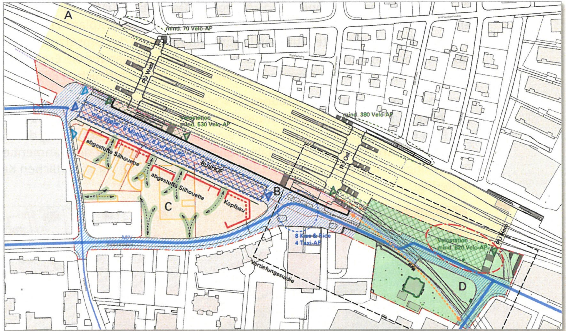
Abb. 3: Entwicklung Bahnhofareal Lenzburg, Syntheseplan, Basler & Hofmann, 2.11.2019
